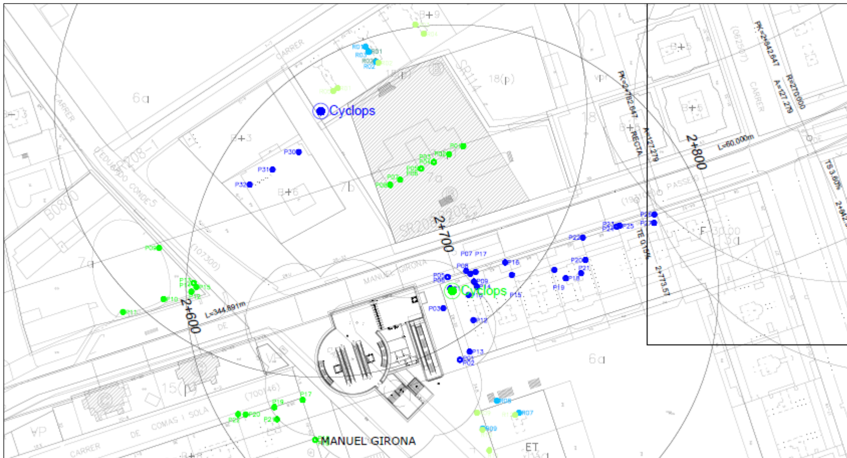
Planta instrumentació d'edificis amb teodolit automàtic
