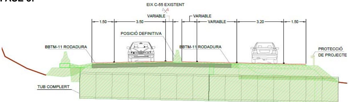
Figura 4. Secció entre el 0+000 i el 2+100 (aprox.)
