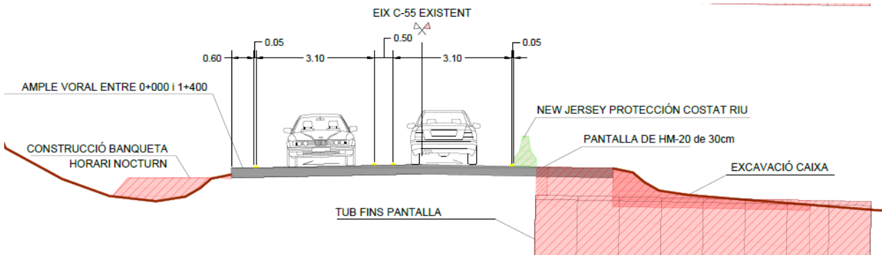
Figura 2. Secció entre el 0+000 i el 1+400 (aprox.)
