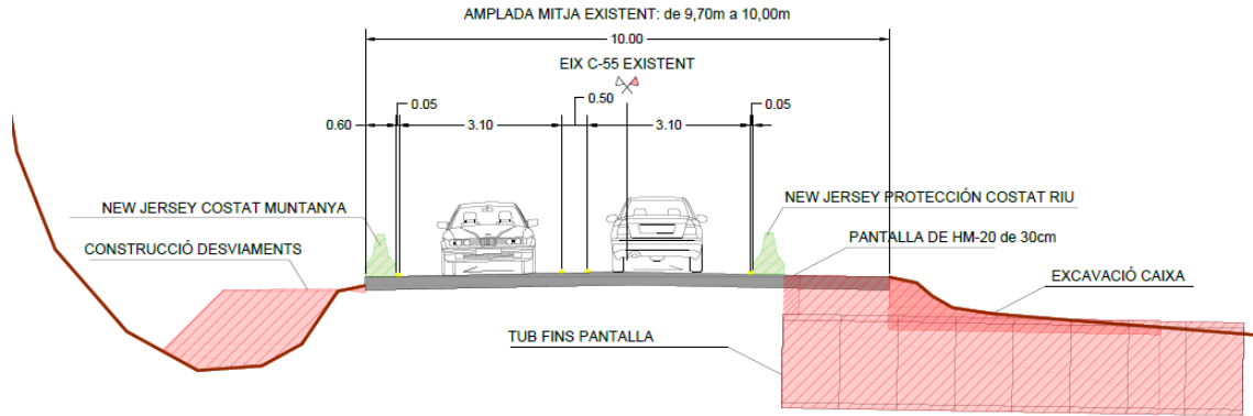
Figura 1. Secció entre el 1+400 i el 2+100 (aprox.)
