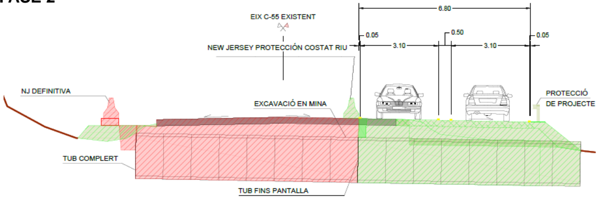
Figura 3. Secció entre el 0+000 i el 2+100 (aprox.)
